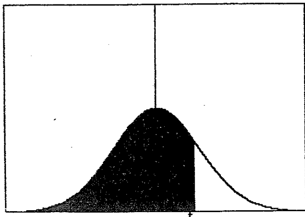
***FUNCION DE DISTRIBUCION DE LA NORMAL (0,1)***
