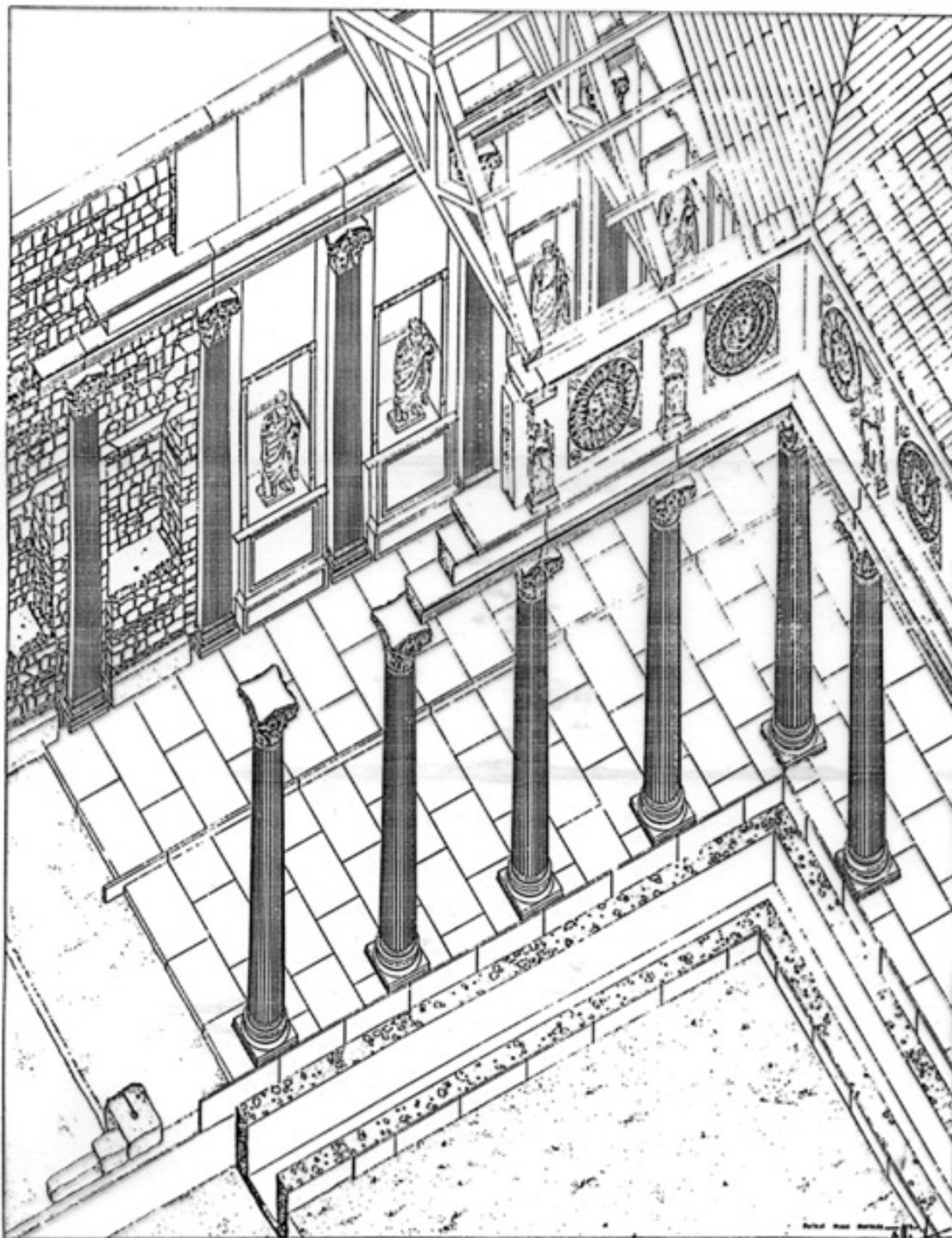
19. Mérida. Sección axonométrica de la reconstrucción ideal del pórtico del Foro Municipal.
