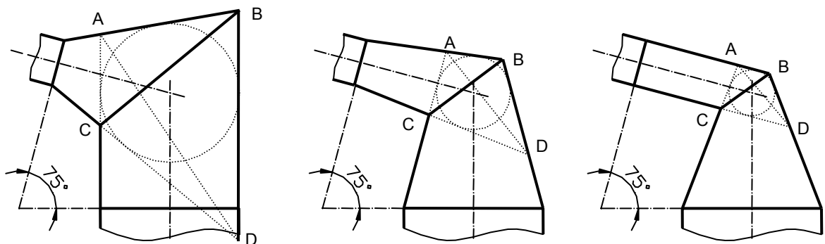
Figura 14. Otras formas de resolución del codo anterior.
