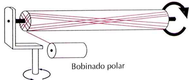
Bobinado circular
