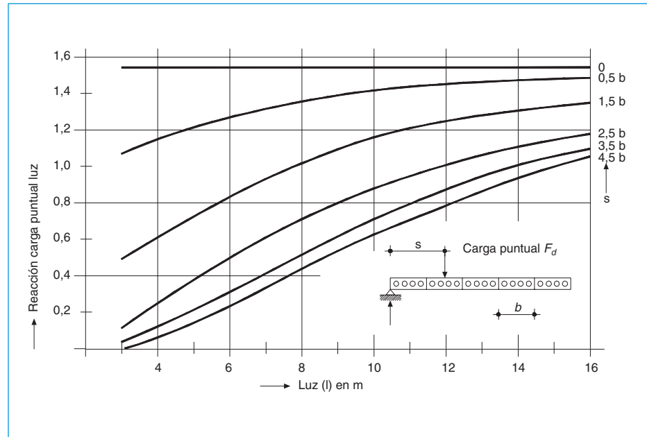
Figura A.12.5.2.5.b Fuerza de reacción en el apoyo longitudinal debida a una carga puntual en el centro de vano ( b = 1,20 \text{ m} )
