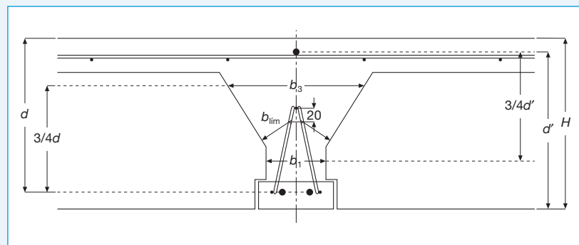
Figura 44.2.1.b. Comprobación de esfuerzo cortante con viguetas armadas
