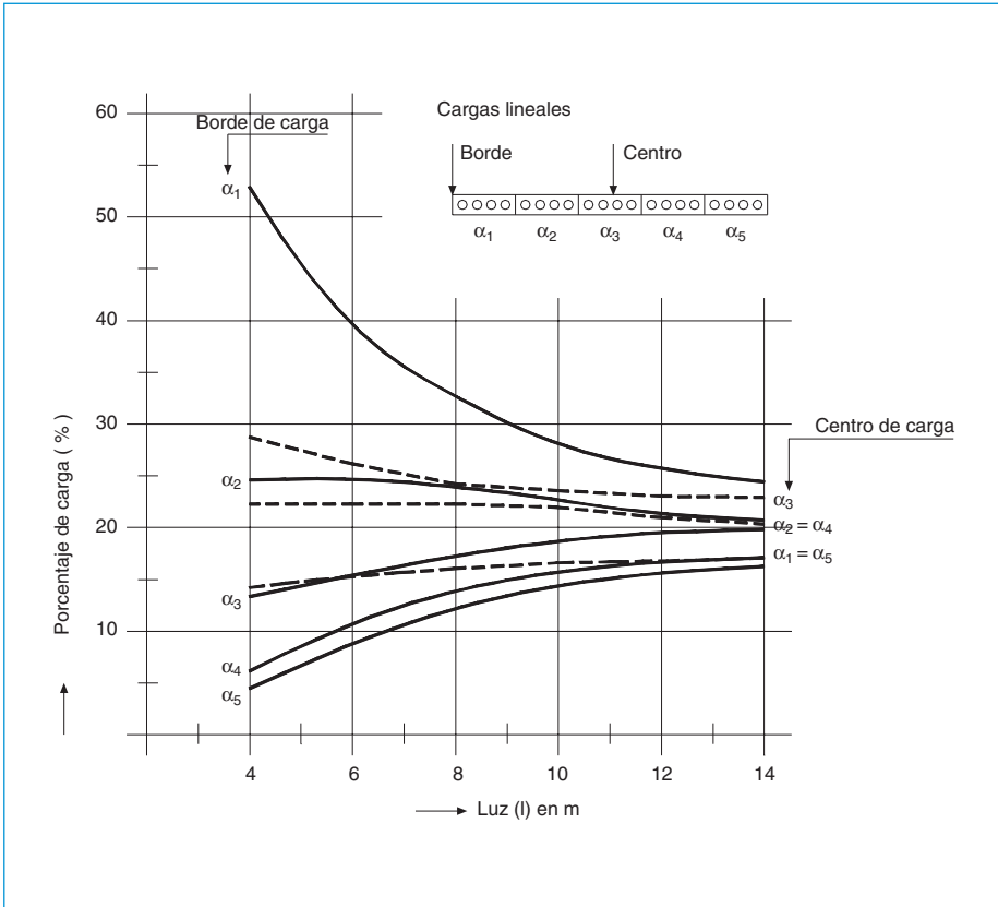
Figura A.12.5.2.4.a Factores de distribución de carga para cargas lineales ( b = 1,20\text{ m} )
