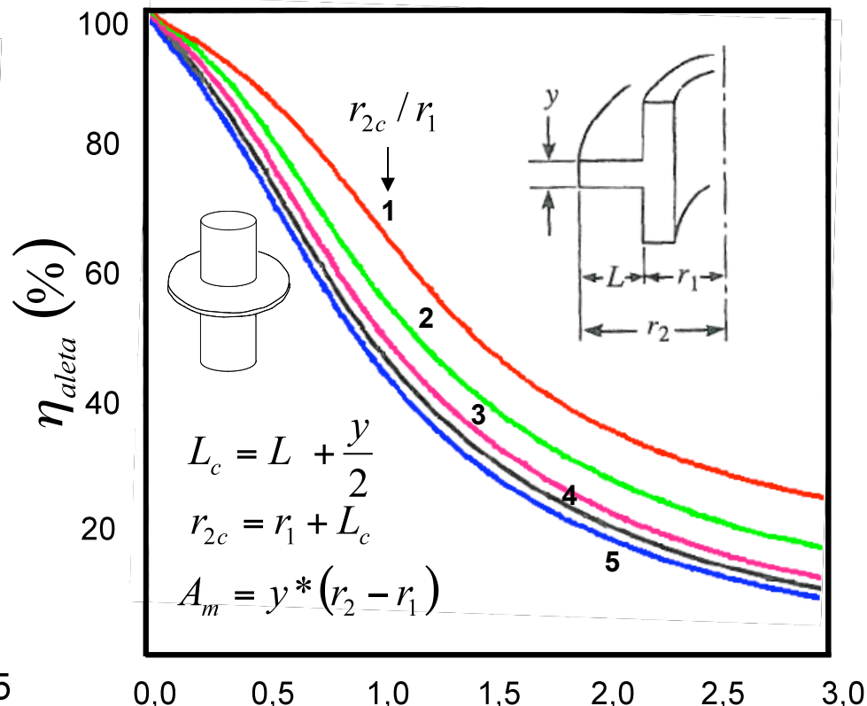
Eficiencia aleta circular
