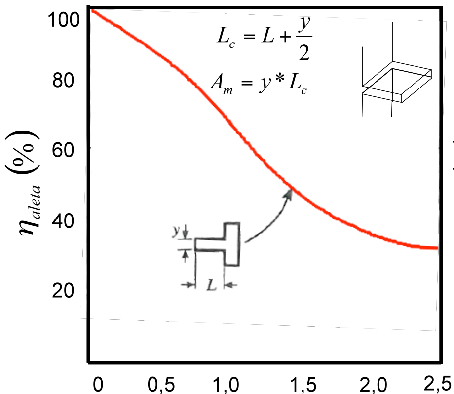
Eficiencia aleta cuadrada
