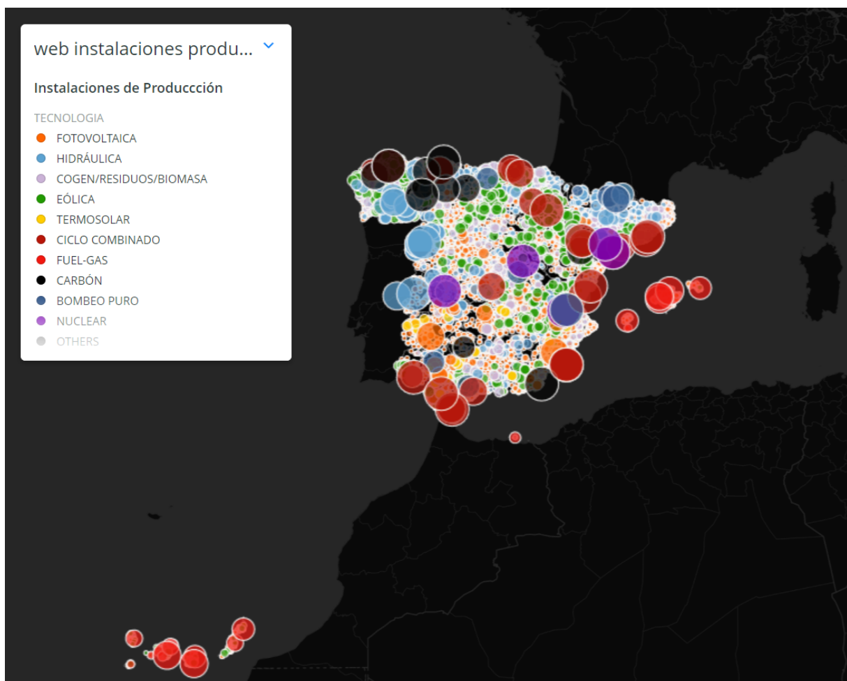
Figura 65. Centrales eléctricas en España (a fecha 2021). Fuente: REE. Enlace: http://bit.ly/30oC8uQ
