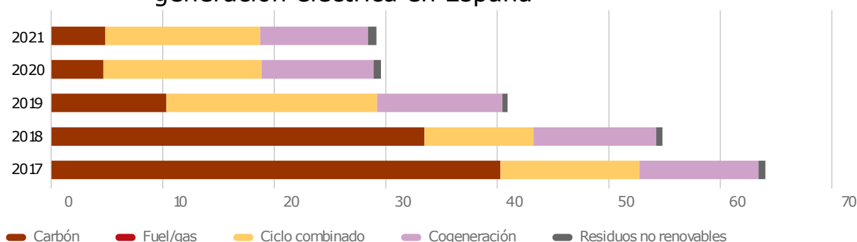
Figura 36. Evolución de las emisiones de CO 2 asociadas con la generación eléctrica en España (finales del 2021). Fuente: REE: “Avance del informe del sistema eléctrico español 2021”. http://bit.ly/2HGg7Ac
