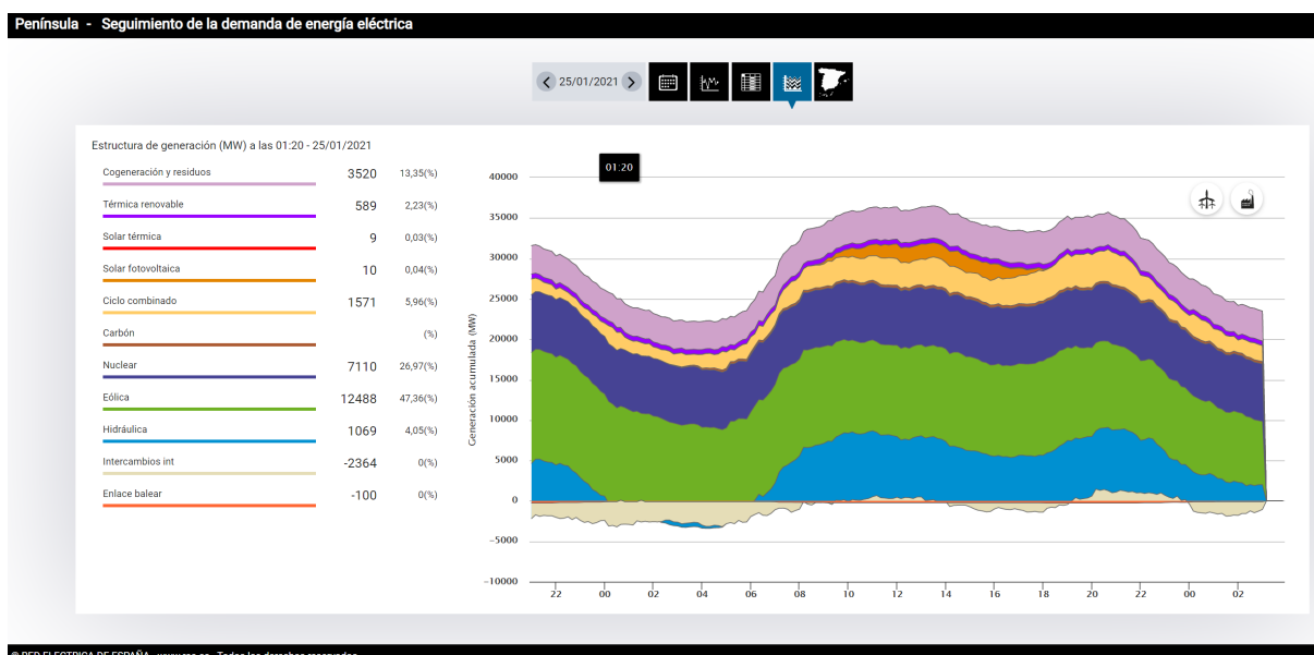
Figura 47. Detalle de la estructura de generación en tiempo real del sistema eléctrica español: 25 Enero, 2021. Fuente: REE. http://bit.ly/2Mns9D2
