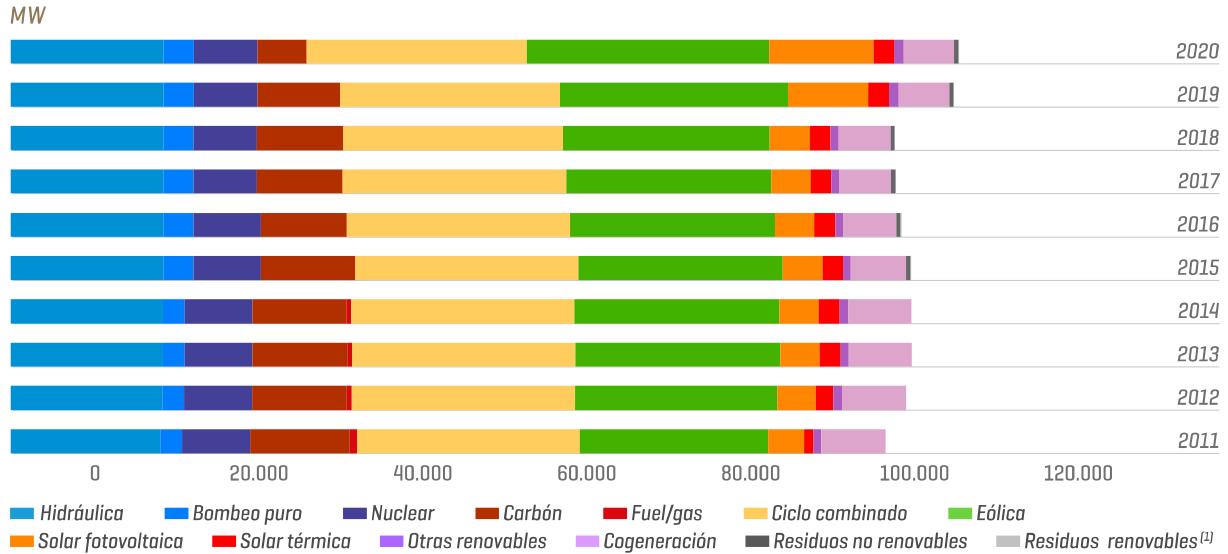
Figura 6. Evolución de la potencia instalada en España (2020). Fuente: “Avance del informe del sistema eléctrico español 2020” https://bit.ly/3mMLITi
