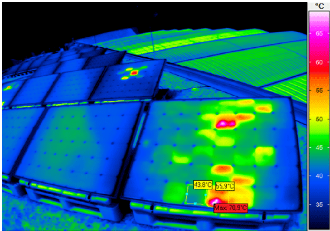
Figura 56. Ejemplo de inspección termográfica de una instalación FV. Fuente: Infratec https://bit.ly/2CDJIok
