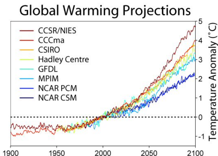
Figura 19. Predicciones sobre la evolución del cambio climático suponiendo un escenario sin reducción de emisiones. Fuente: Global Warming Art. Licencia CC BY-SA 3.0 https://bit.ly/2JI5j3j
