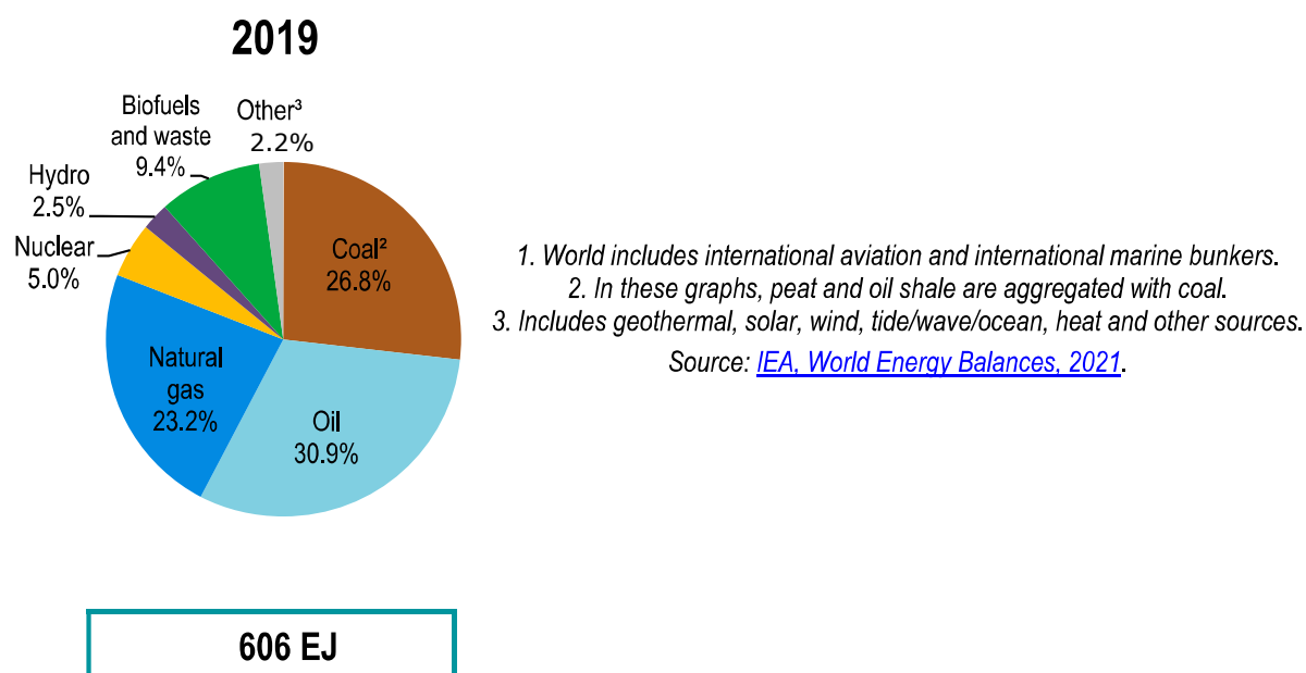
Figura 1. Contribuciones a la demanda de energía primaria global (2019). Fuente: Key world energy statistics 2021. Enlace: https://bit.ly/3IU3nTQ
