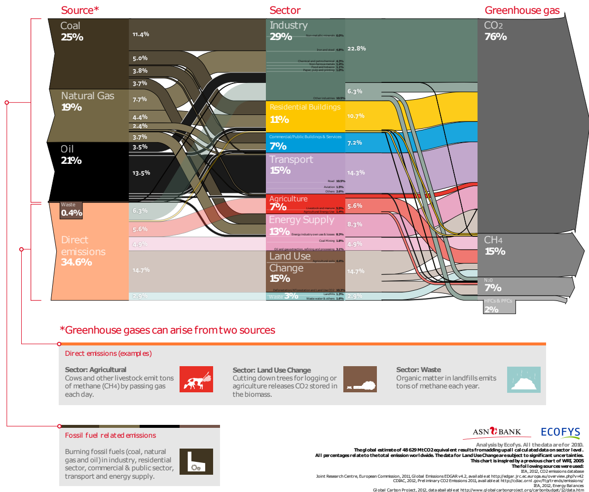
Figura 20. Diagrama de flujo de las emisiones mundiales de gases de efecto invernadero. Fuente: ECOFYS. http://bit.ly/2AwkICXk
