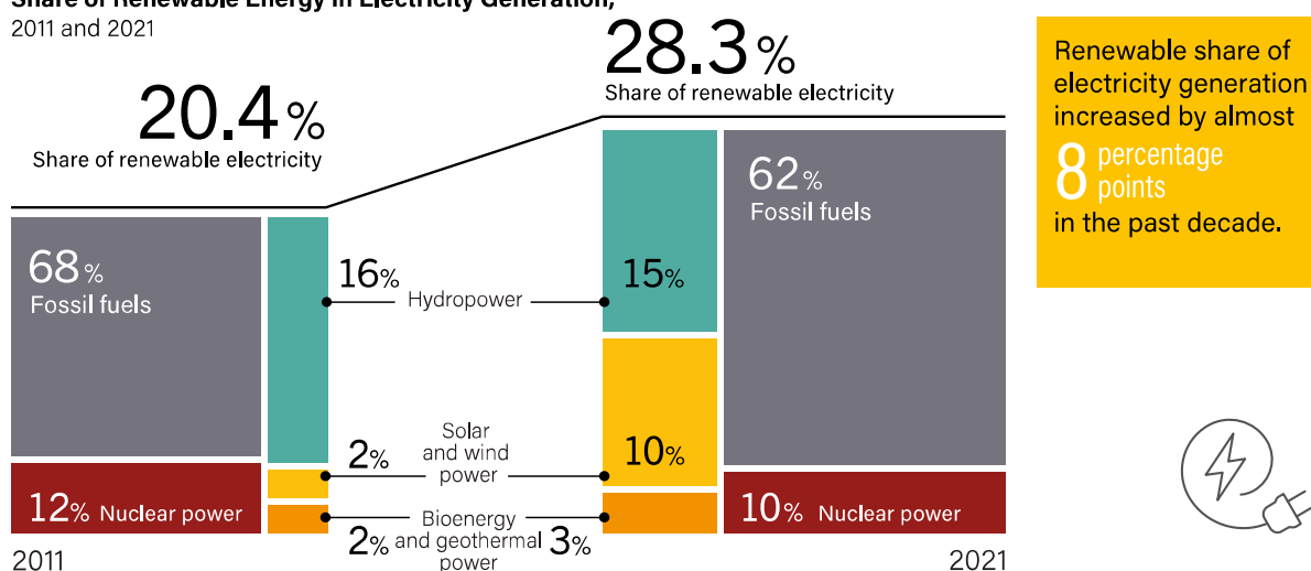
Figura 24. Cobertura de las EERR en relación al consumo global de energía eléctrica (final-2021). Fuente: REN21 (2022 Report). Enlace: https://bit.ly/3MR1R7x .
