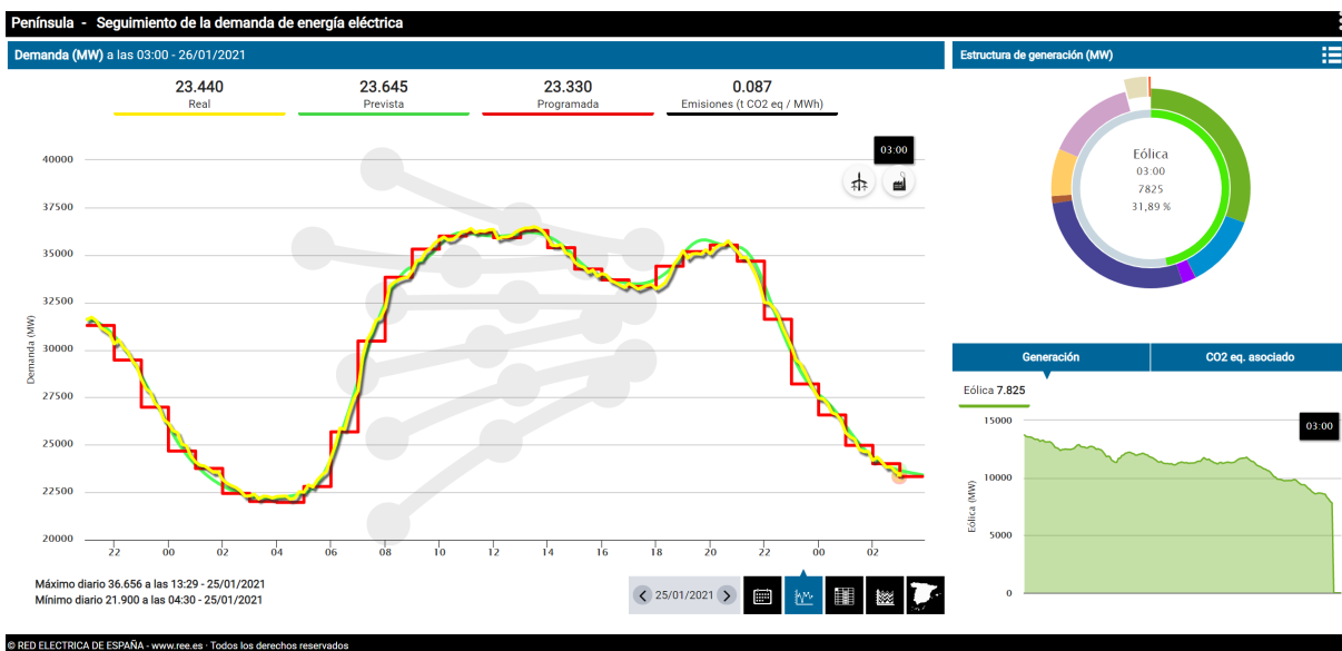
Figura 46. Ejemplo de información en tiempo real sobre demanda y generación en el sistema eléctrica español: 25 Enero, 2021). Fuente: REE. http://bit.ly/2Mns9D2
