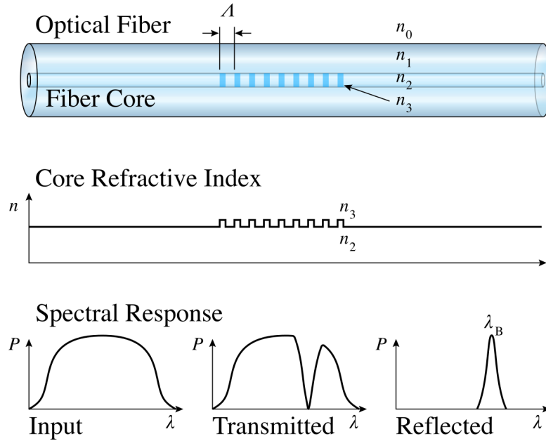
Figura 59. Esquema del funcionamiento de un FBG. Fuente: Wikimedia Commons. Licencia: CC BY-SA 3.0. http://bit.ly/2JDIjGJ
