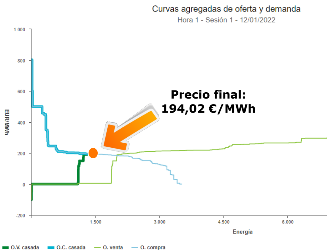
Figura 45. Ejemplo de subasta de electricidad (12 de enero de 2022). Curvas de oferta y demanda (órdenes de compra y venta en marrón y azul, respectivamente). Fuente: OMIE http://omie.es
