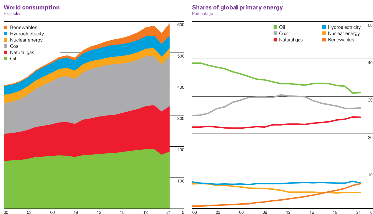
Figura 12. Evolución del consumo de energía mundial según la fuente empleada. Fuente: BP Statistical Review of World Energy 2022. Enlace: https://on.bp.com/3MQk8q
