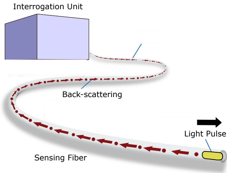
Figura 61. Esquema del principio de funcionamiento de los sensores distribuidos de fibra óptica basados en procesos de scattering. Fuente: YouTube. Licencia: YouTube standard. https://youtu.be/TQmtv45D50A .
