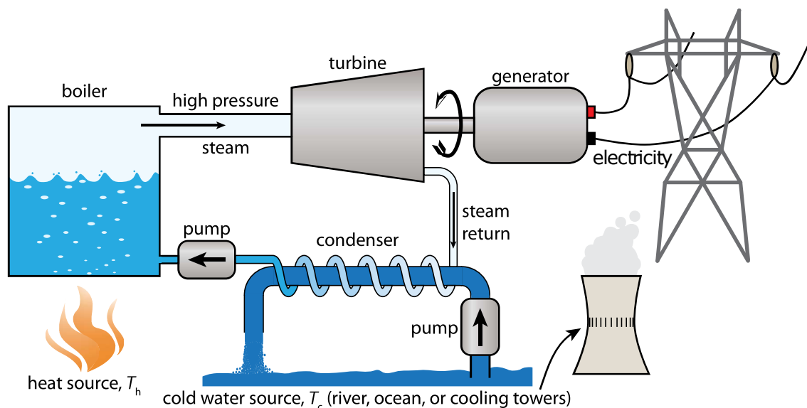
Figura 5. Esquema de funcionamiento de una planta de generación eléctrica genérica. Fuente: “Energy and human ambitions on a finite planet” (Thomas W. Murphy). Licencia: CC-by-NC 4.0. Enlace: https://bit.ly/3d0Rg9N .
