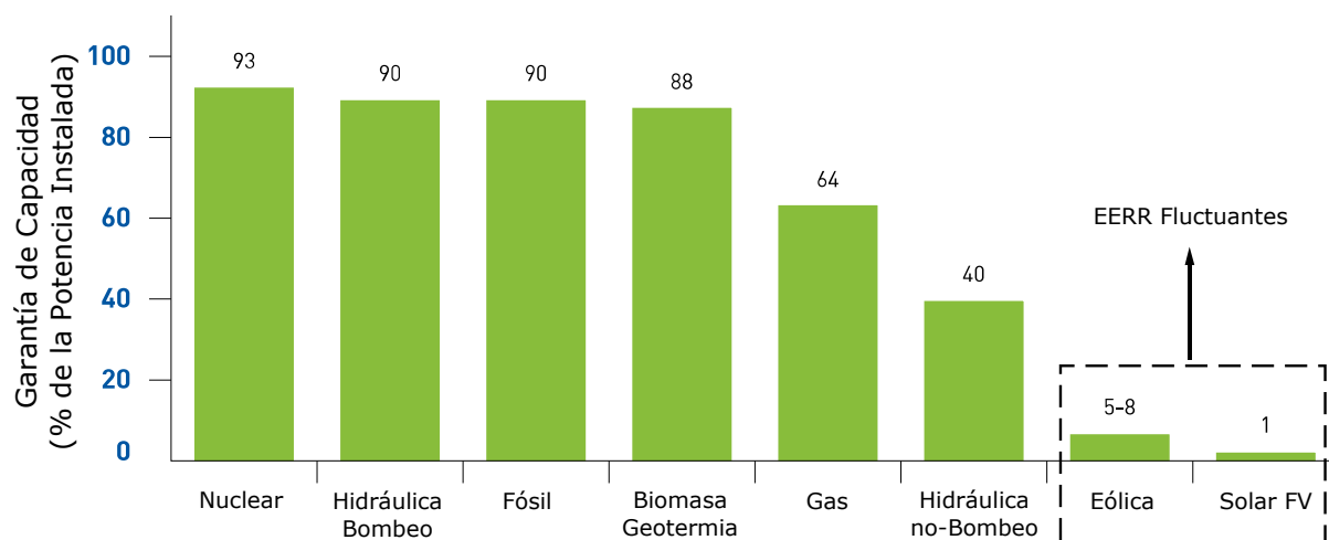
Figura 48. Garantía de capacidad asociada a diferentes tecnologías de generación eléctrica. Fuente: IDAE ( Evolución tecnológica y prospectiva de costes de las EERR ). http://bit.ly/2nRALmR
