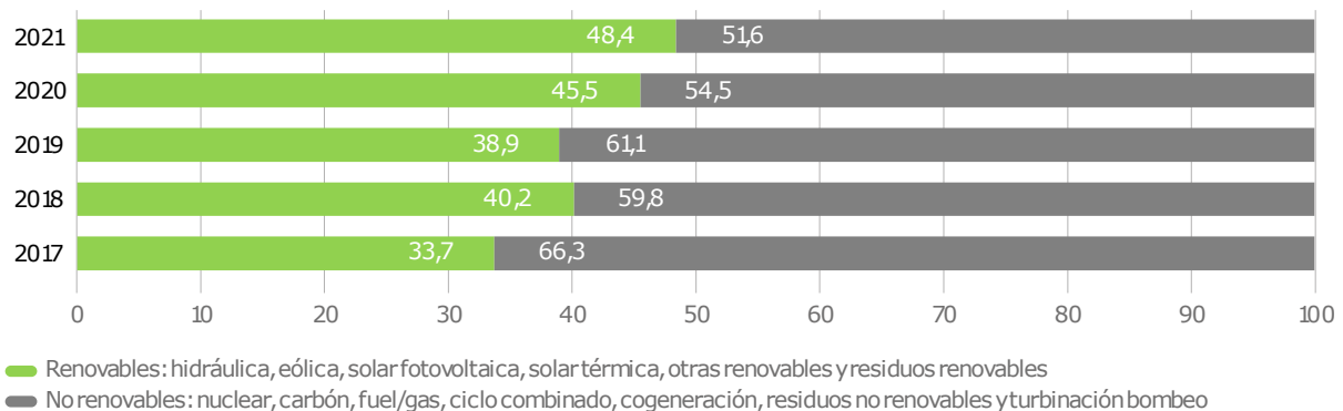
Figura 34. Evolución de la contribución de fuentes renovables y no-renovables (2021). Fuente: REE: “El sistema eléctrico español: previsión de cierre 2021” . https://bit.ly/3oalRUI
