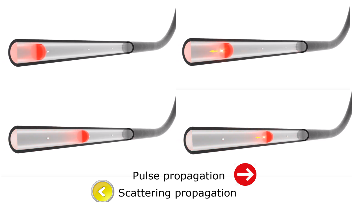
Figura 62. Esquema del principio de funcionamiento de los sensores distribuidos de fibra óptica basados en procesos de scattering (detalle de la unidad interrogadora). Fuente: fibergratings.com. http://bit.ly/2HHCyWu .
