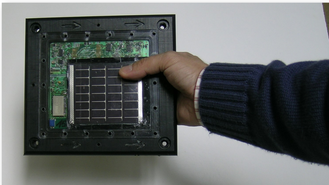
Figura 55. Sistema de aforo automático desarrollado por el Grupo de Ingeniería Fotónica de la Universidad de Cantabria.
