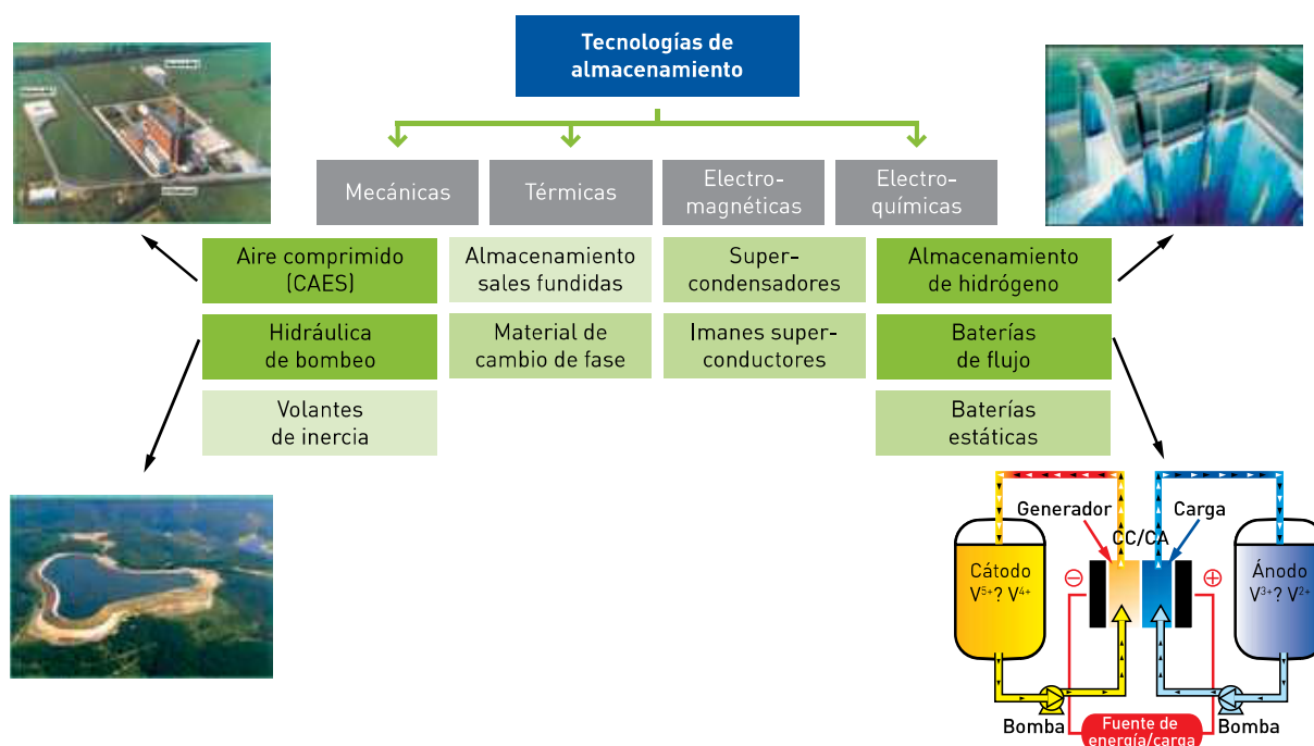
Figura 49. Tecnologías de almacenamiento de energía en la red eléctrica. Fuente: IDAE ( Evolución tecnológica y prospectiva de costes de las EERR ). https://bit.ly/2nRALmR
