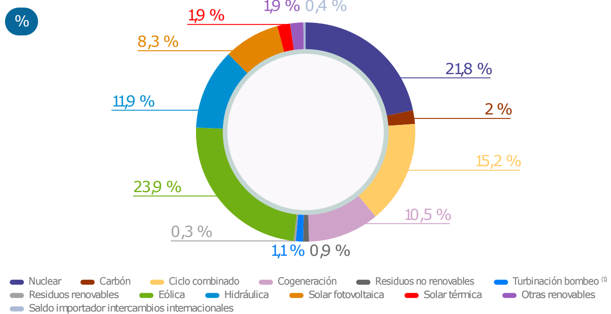
Figura 8. Generación eléctrica en España (2021). Fuente: REE: “Avance del informe del sistema eléctrico español 2021”. http://bit.ly/2HGg7Ac
