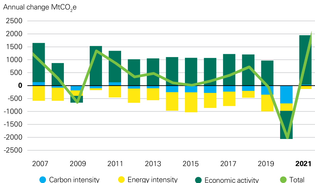
Figura 21. Evolución de las emisiones de CO 2 hasta 2021. Fuente: Statistical Review of World Energy 2022. Enlace: https://on.bp.com/3MOQk8q
