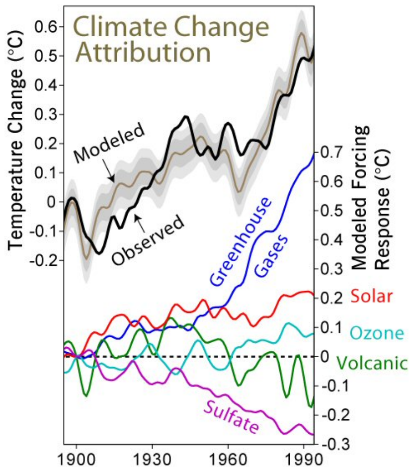
Figura 18. Modelos de la evolución de la temperatura media de la superficie de la Tierra. Fuente: NASA. Licencia CC BY-SA 3.0 https://bit.ly/2BWnopk
