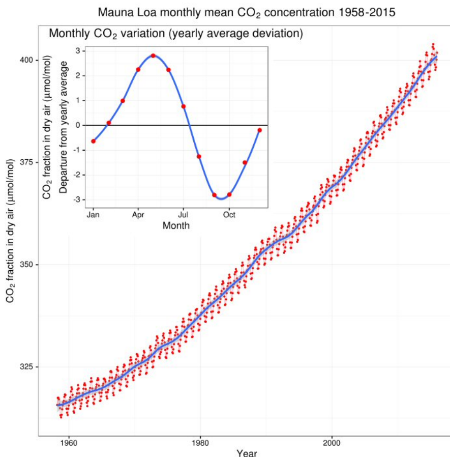
Figura 17. Evolución de los niveles de CO 2 medidos en la isla de Mauna Loa (Hawái) ( Keeling Curve ). Fuente: Delorme - Own work. Data from Dr. Pieter Tans, NOAA/ESRL and Dr. Ralph Keeling, Scripps Institution of Oceanography. Licencia CC BY-SA 4.0. https://bit.ly/2yZvyyM
