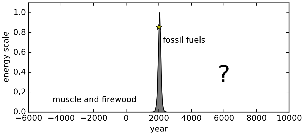
Figura 9. Uso de los combustibles fósiles a lo largo del tiempo. Fuente: “Energy and human ambitions on a finite planet” (Thomas W. Murphy). Licencia: CC-by-NC 4.0. Enlace: https://bit.ly/3d0Rg9N .
