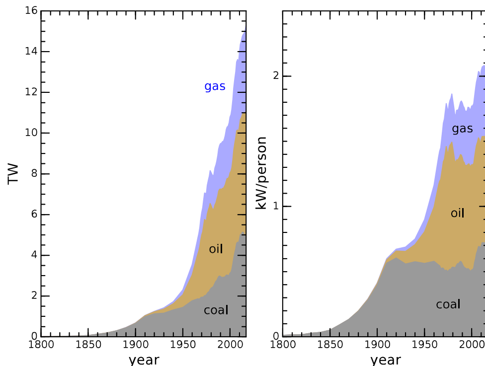
Figura 10. Uso de combustibles fósiles desde la Revolución Industrial. Fuente: “Energy and human ambitions on a finite planet” (Thomas W. Murphy). Licencia: CC-by-NC 4.0. Enlace: https://bit.ly/3d0Rg9N .
