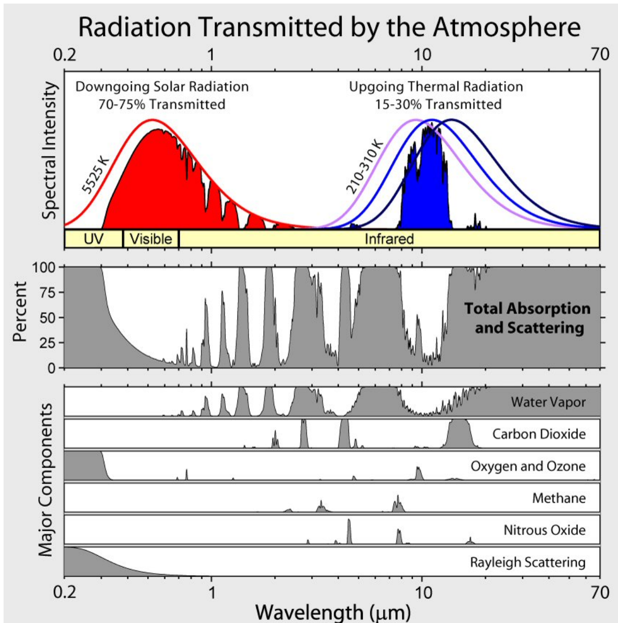
Figura 15. Radiación transmitida por la atmósfera terrestre (radiación entrante (rojo) y saliente (azul)). Fuente: https://bit.ly/2JNVJfe
