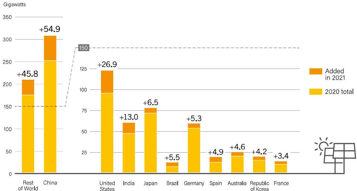
Figura 29. Potencia solar FV de los 10 países líderes y potencia añadida en 2021. Fuente: REN21 (2022 Report). Enlace: https://bit.ly/3MR1R7x .
