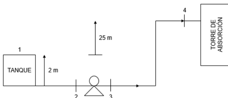
Figura 1. Diagrama de proceso.
